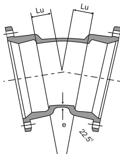
زانوئی دو سر ساکت ۲۲/۵ درجه (بولتد گلند)
