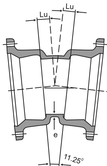
زانوئی دو سر ساکت ۱۱/۲۵ درجه (بولتد گلند)
